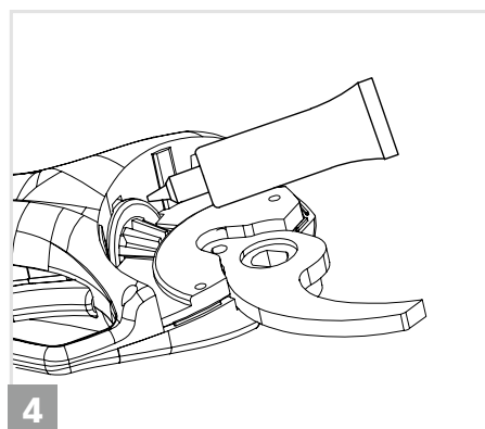
4. Auf die Zahnradzähne und den Zentrierbolzen Schmierfett auftragen. Den gleichen Vorgang ausführen, auch wenn die Klinge durch eine neue Klinge ersetzt wird.
